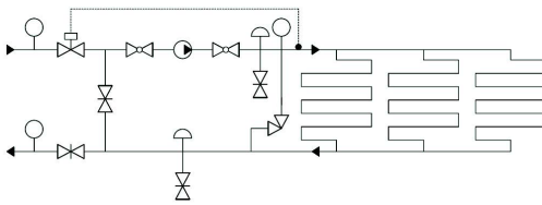
ГИДРАВЛИЧЕСКАЯ СХЕМА УЗЛОВ С РЕГУЛИРОВКОЙ ТЕМПЕРАТУРЫ С ФИКСИРОВАННЫМ ЗНАЧЕНИЕМ
