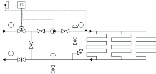
ГИДРАВЛИЧЕСКАЯ СХЕМА УЗЛОВ С УПРАВЛЕНИЕМ ВНЕШНИМ КОНТРОЛЛЕРОМ
