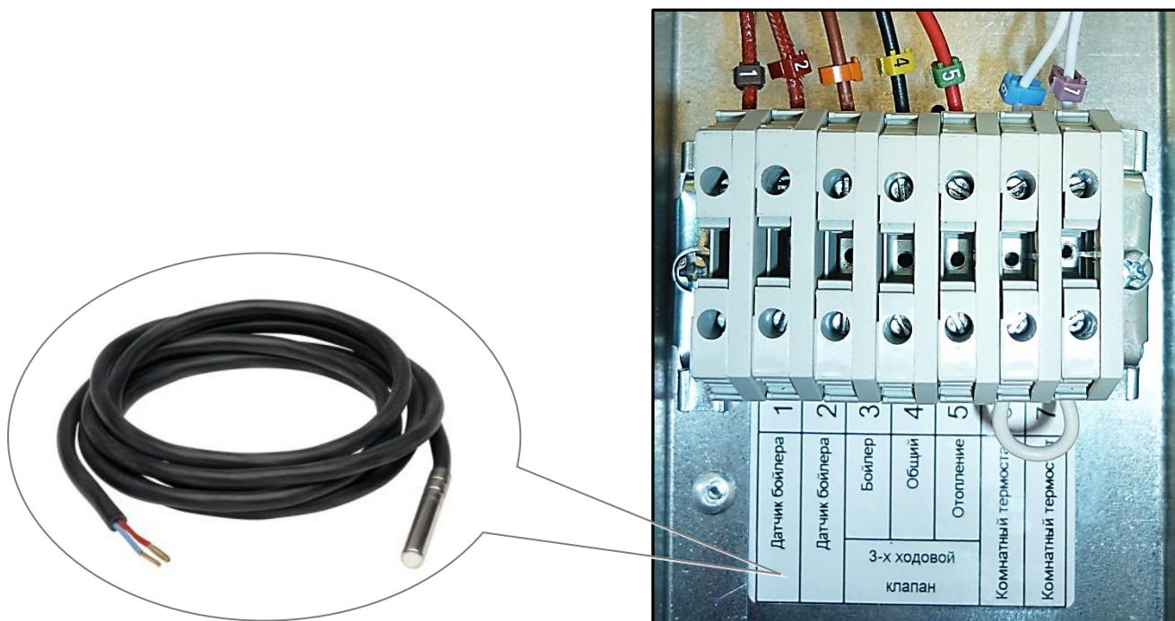
Рис.24 Подключение датчика температуры бойлера трёхходового клапана «ARDERIA» к клеммной колодке.
