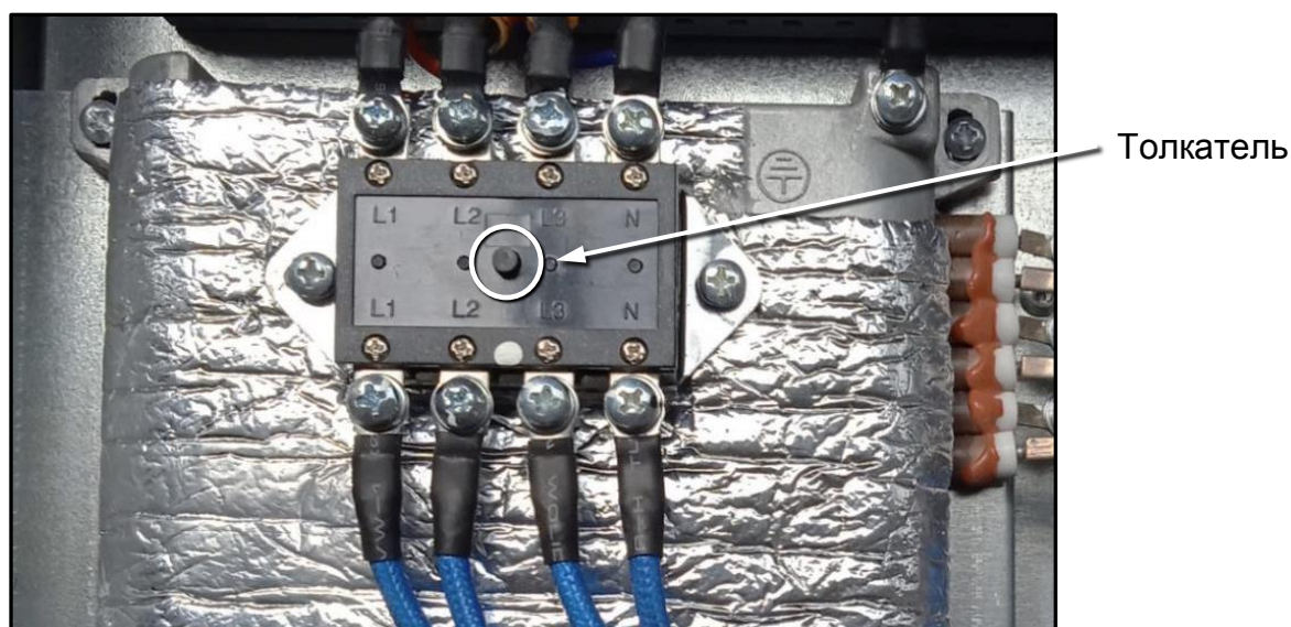
Рис. 8 Силовой биметаллический термостат (датчик перегрева)
