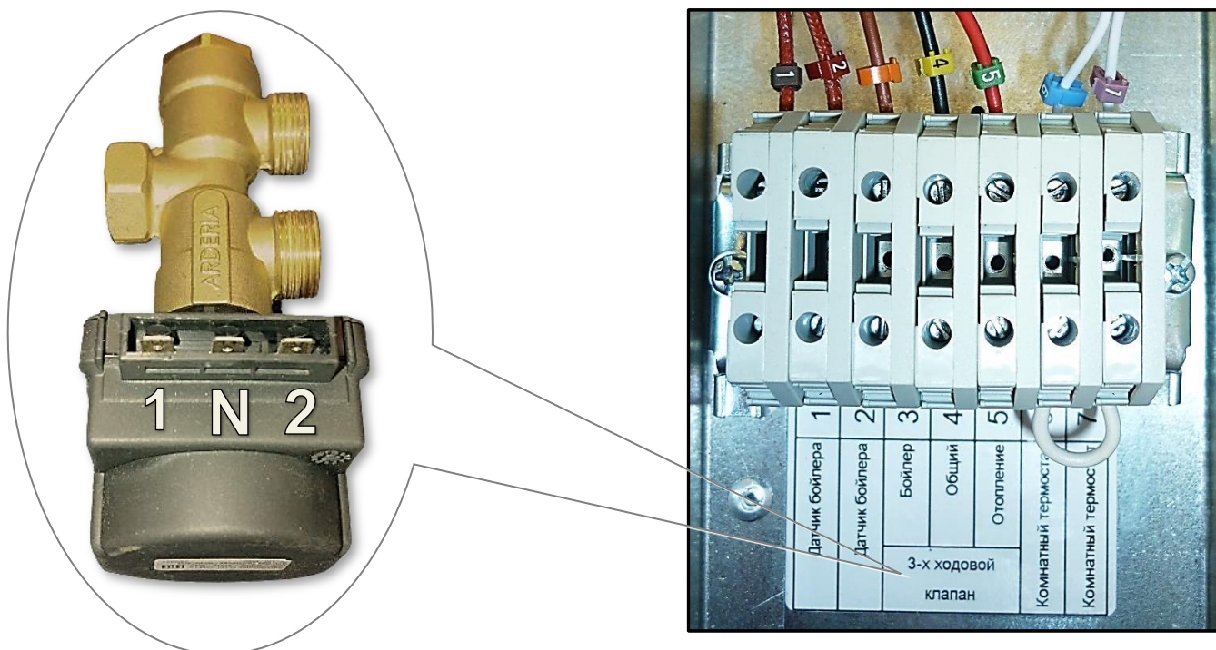
Рис.23 Подключение трёхходового клапана «ARDERIA» к клеммной колодке.
