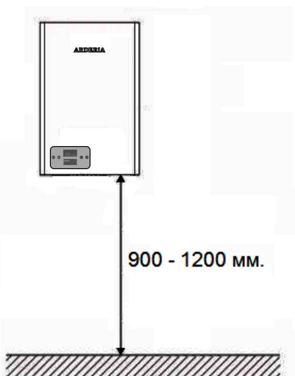
Рис. 10 Монтажные расстояния
