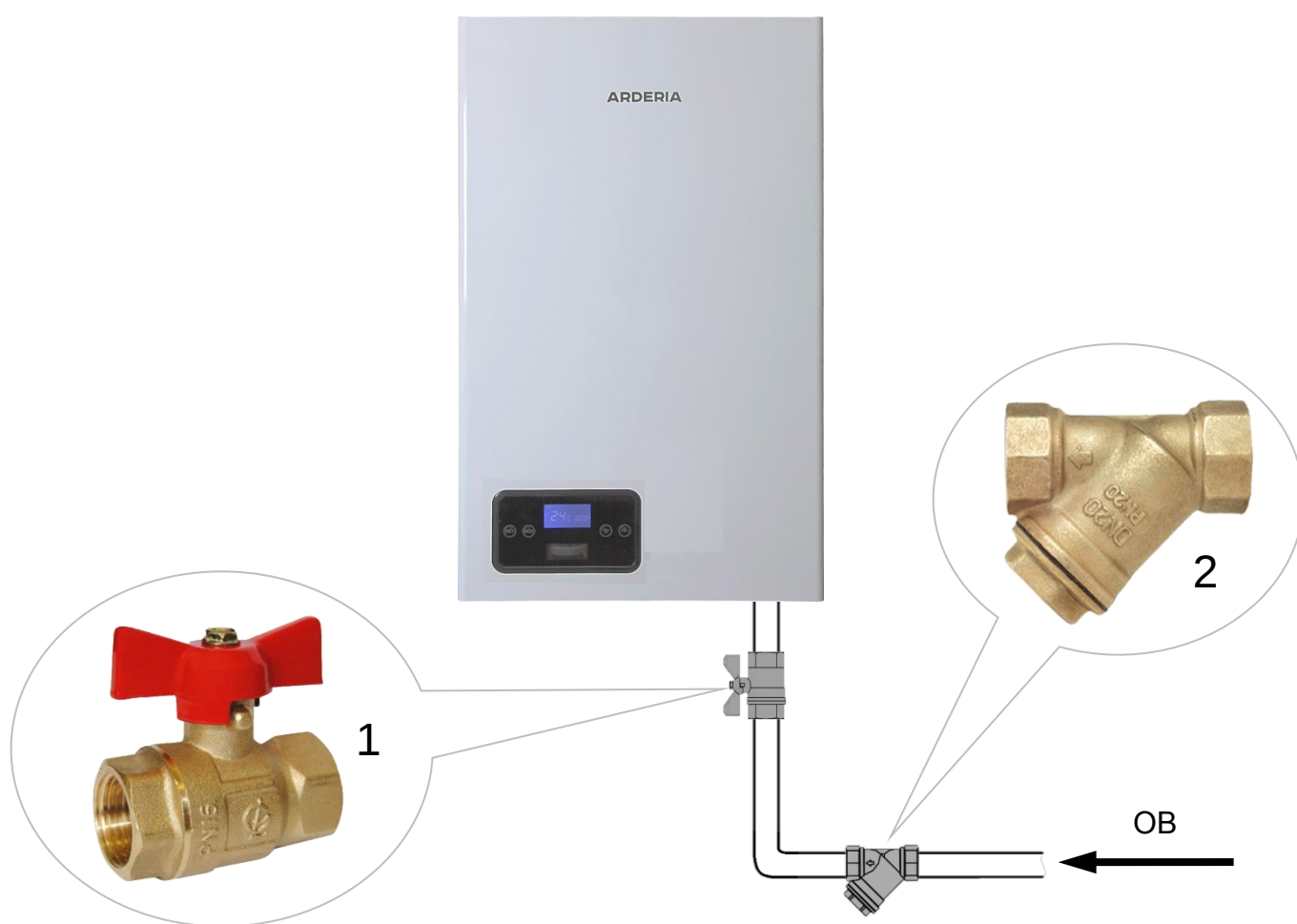
Рис. 19 Монтаж труб системы отопления
