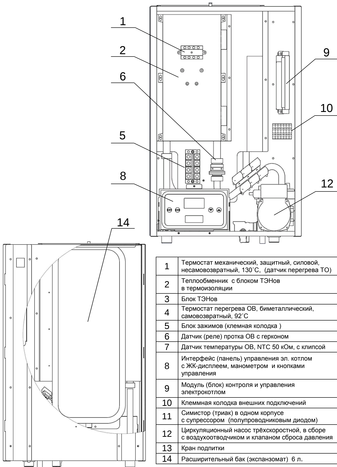
Рис. 2 Внутренне устройство
