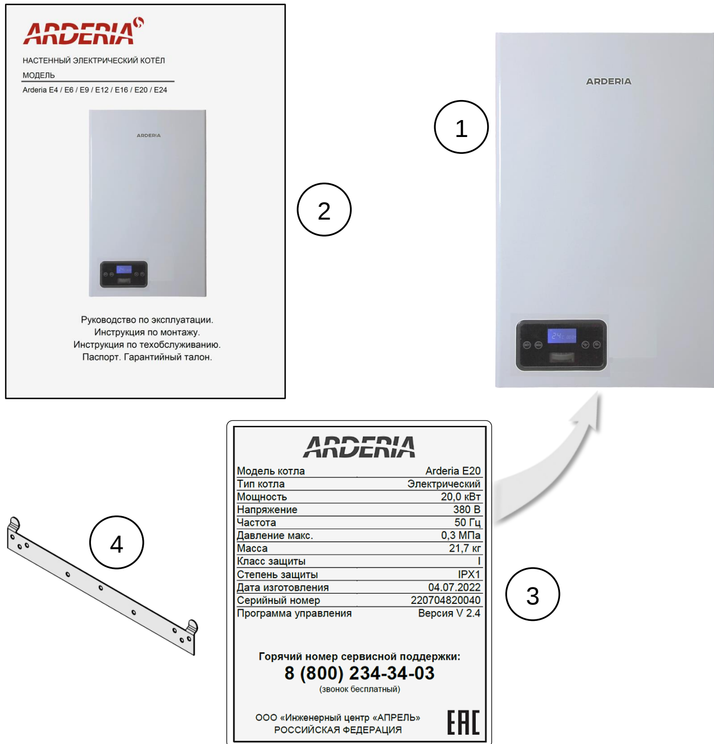
Рис. 4 Комплект поставки
