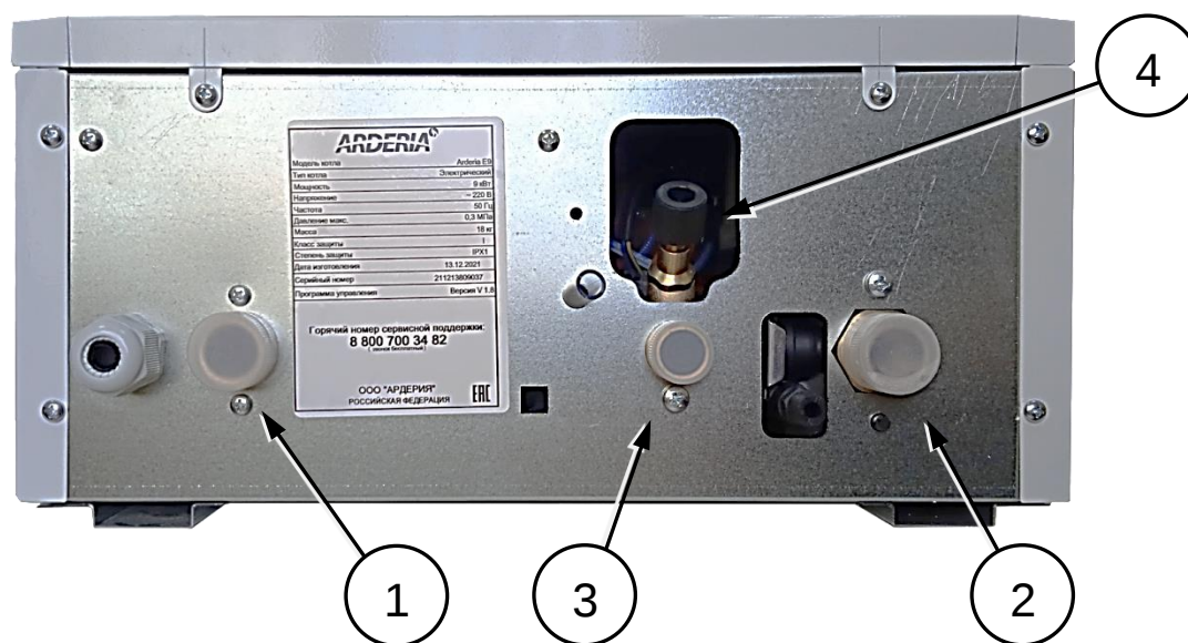
Рис. 18 Патрубки присоединения электрокотла к трубам
