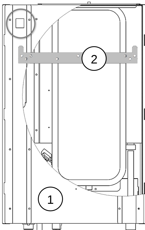
Рис. 12 Монтажные отверстия электрокотла
