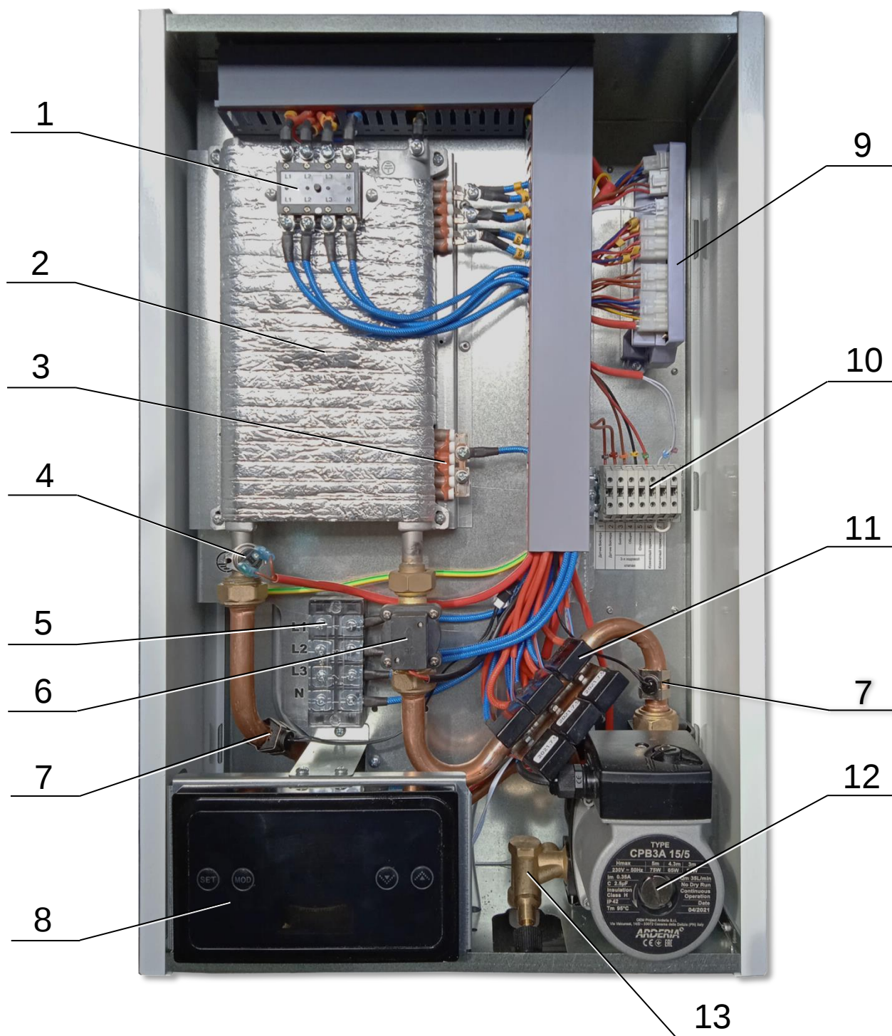
Рис. 1 Общий вид
