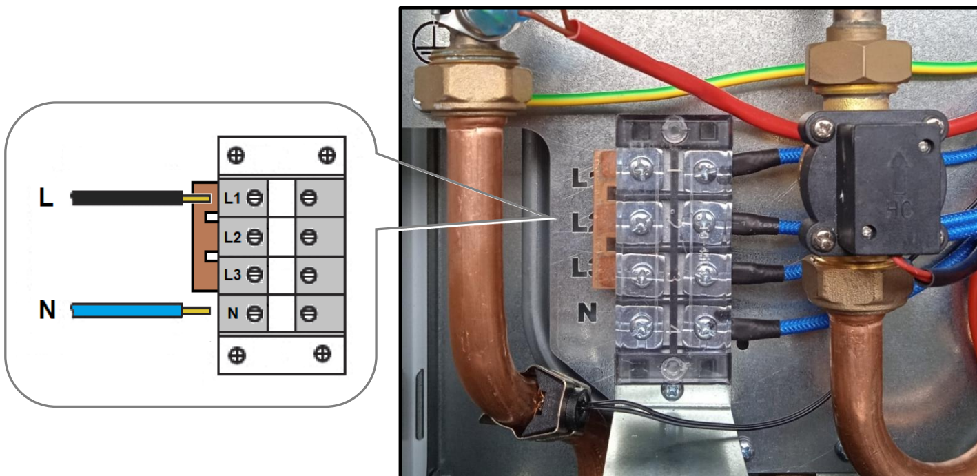
Рис. 15 Однофазное подключение
