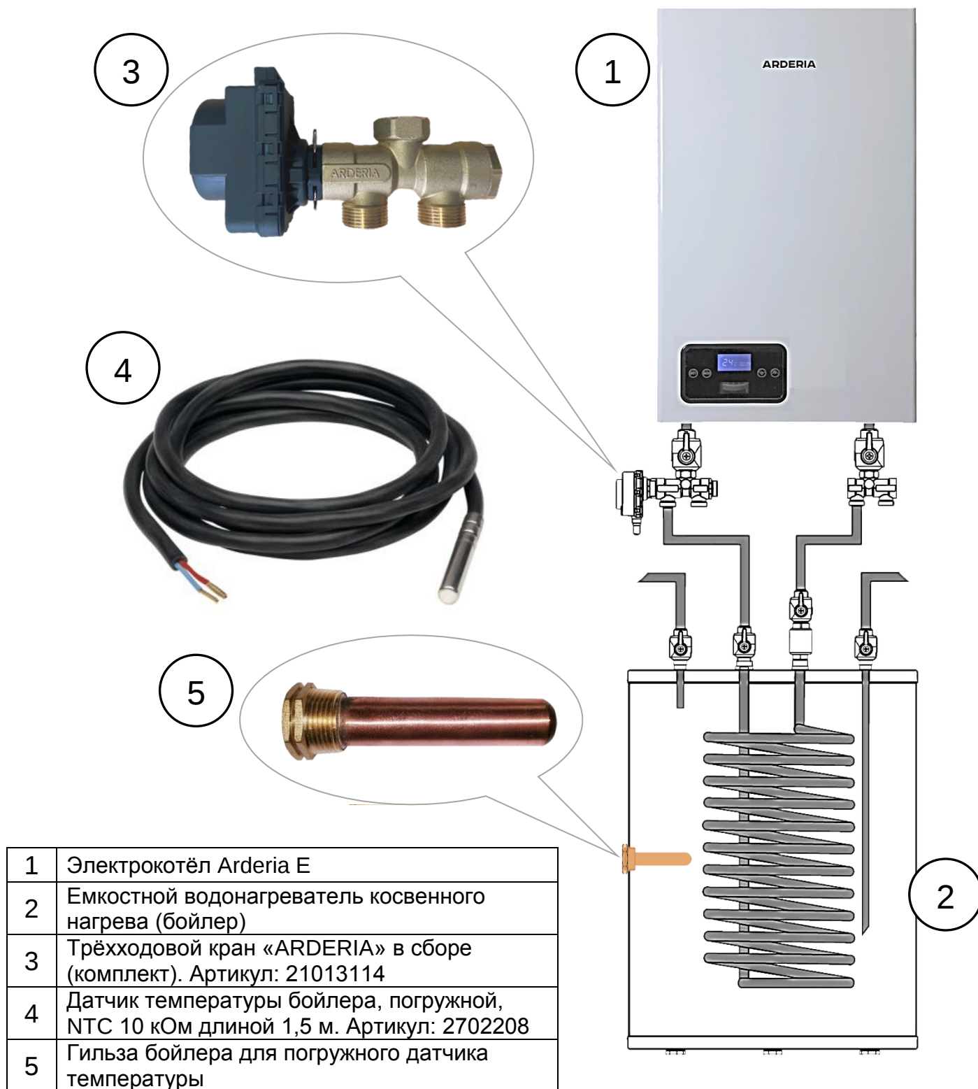
Рис. 22 Принципиальная монтажная схема подключения электрокотла к ёмкостному водонагревателю косвенного нагрева (бойлеру)
